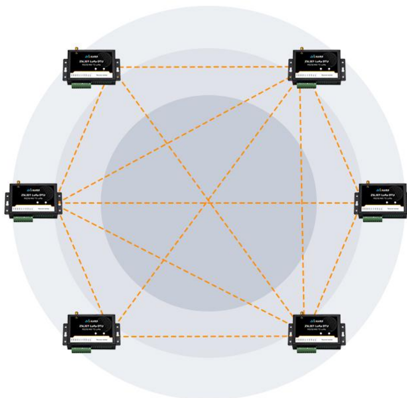
Mesh网拓扑图
